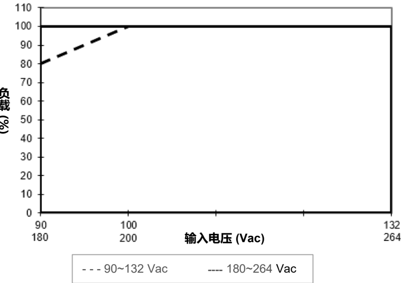
图 2 AC 输入电压降额 < 100 Vac 功率降额 2% / V (80% 负载 @ 90 Vac)
