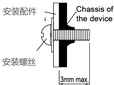
图 4 安装螺丝
