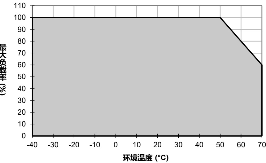
图 1 水平安装降额 > 50°C 功率降额 2.0% / °C
