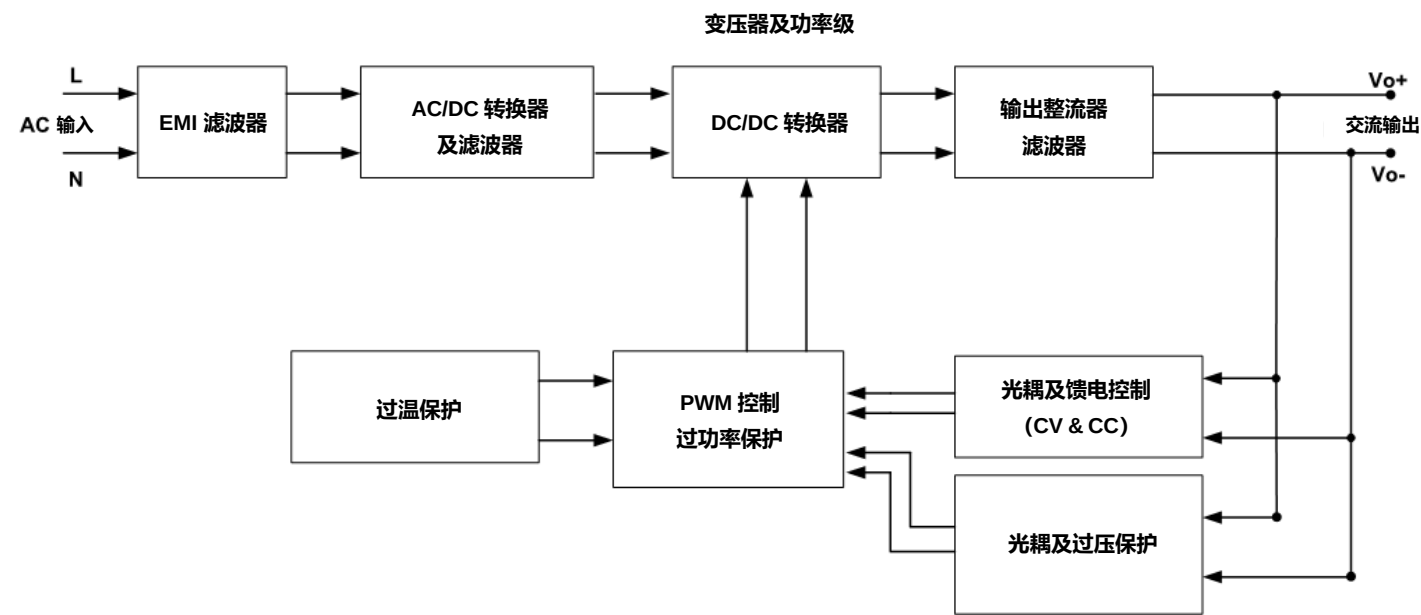
方块图
