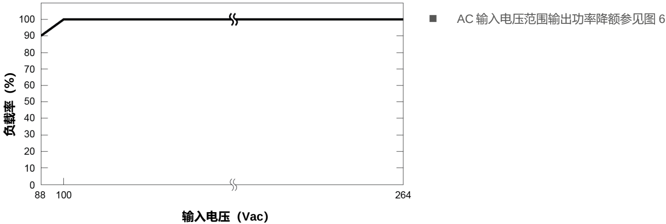
图. 6 AC 输入电压降额 < 100 Vac 功率降额 0.83% / V
