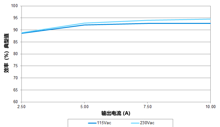
图. 2 效率对比输出负载 (24 V 输出)
