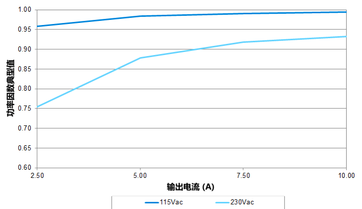
图. 4 功率因数对比输出负载 (24 V 输出)
