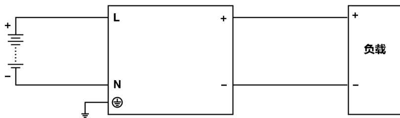
图. 13 DC 输入模式连接电路图
