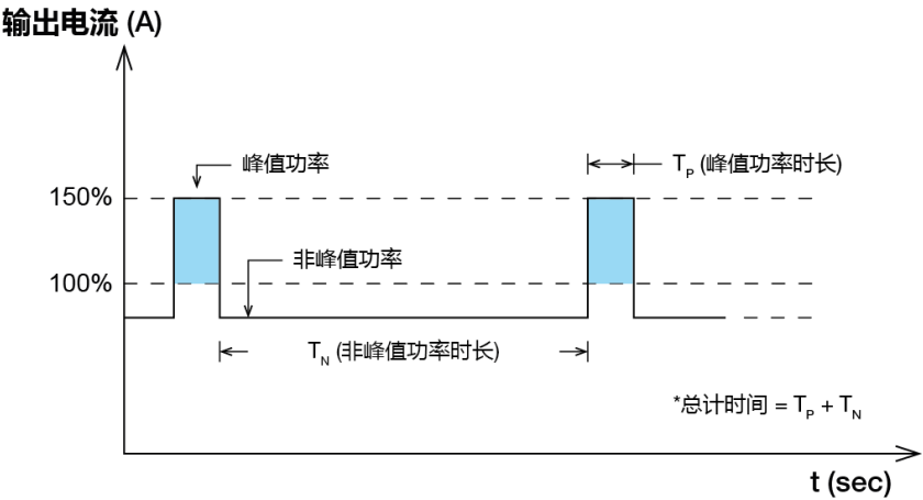
图. 8 占空比计算
