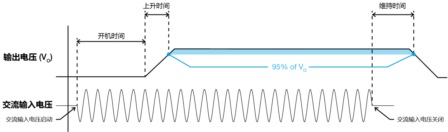
■ 开机时间、上升时间及维持时间图表
