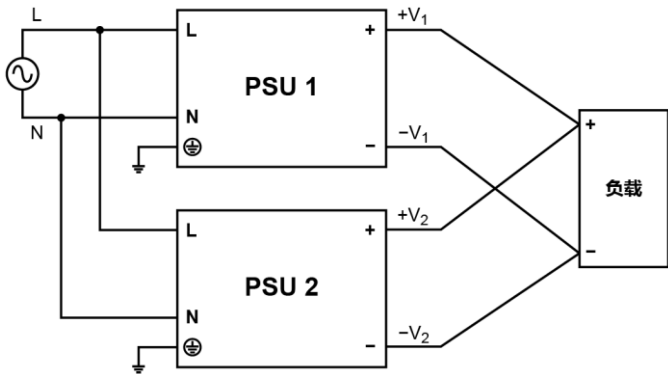
图. 11 并联模式连接电路图
