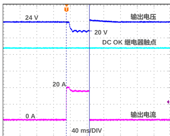
图. 9 APB 200% 额定输出电流持续 50 ms
