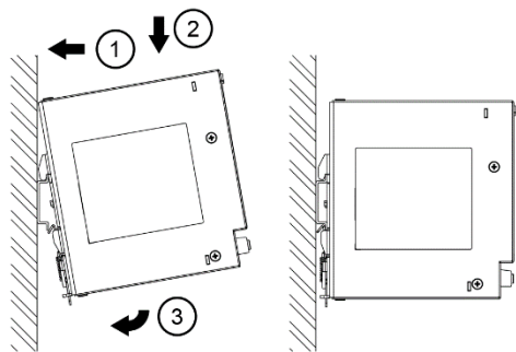
图. 7.1 安装
