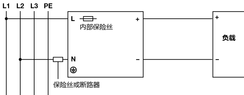
图. 14 三相系统的两相输入运行电路图
