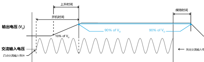
图 5. 时间顺序
