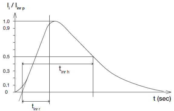
图 7. 浪涌电流
