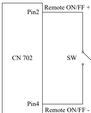
图 9. 遥控 On/Off 连接示意图
