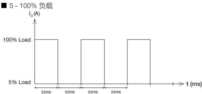
图 6. 动态负载
