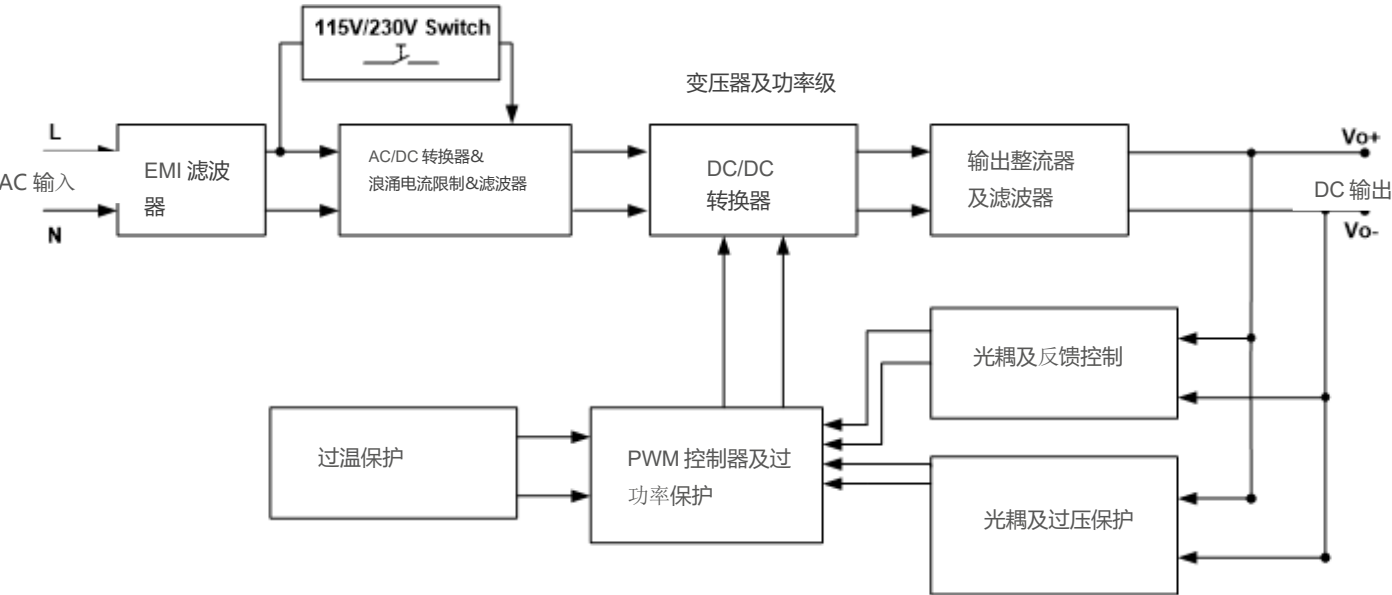
方块图
